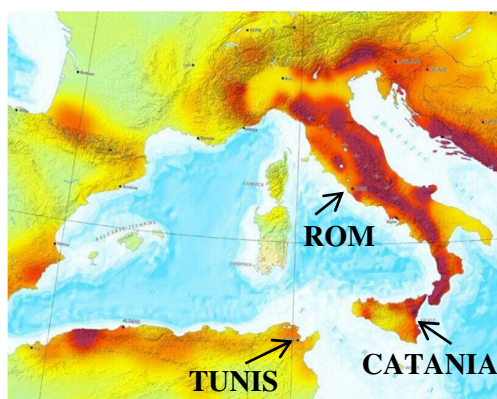
Abb.1: Erdbebengefährdungskarte Europa
